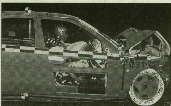
Gyűrődési zónák: Tompítják az első és hátsó ütközéseket.
