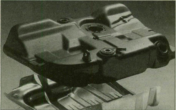
Ütközésbiztos üzemanyagtartály: Csökkenti a kigyulladás veszélyét.
