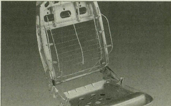
Kicsúszást gátló ülések: Ütközéskor megtartják a testet.
