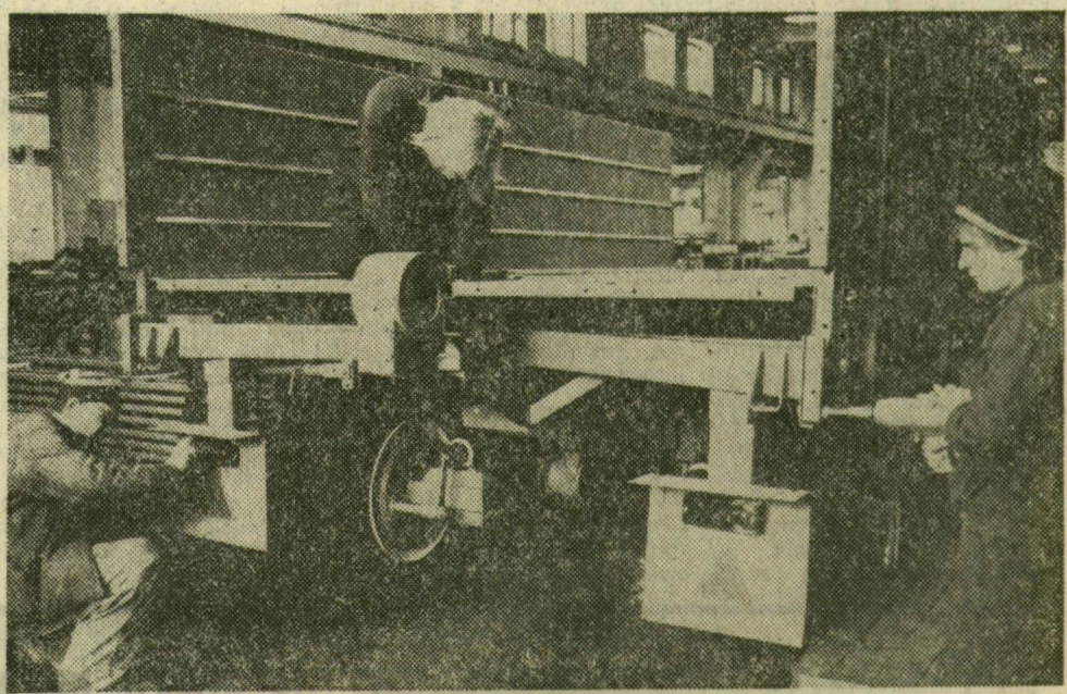
Nagy László felvétele. Államközi szerződés keretében készülnek a T-098-as pótkocsik a Hódgép dorozsmai gyáregységében. Tavaly 1400 darabot szállítottak belőle az NDK-ba
