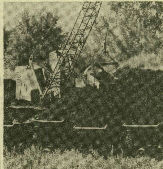
Inota és Nádaslady között az öslábjó havi 6-8 ezer tonna főzeget termelnek ki. Ezt az erősen kötött talajok javítására, a kertészetekben és a gombatenyészetekben használják fel
