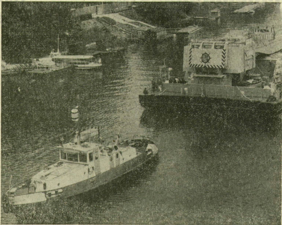
A Magyar Hajó- és Darugár angyalföldi gyáregységében készülnek az úszódaruk. Az idén tizenhat és huszonöt tonna teherbírású folyami, illetve tengeri darukat gyártanak, a Szovjetunió, Románia és Csehszlovákia részére. Az év végéig összesen tizenhét daru készül, ebből az első félévben a tervezettnél eggyel többet adták át a megrendelőnek. Képünkön: útjára indul az úszódaru
