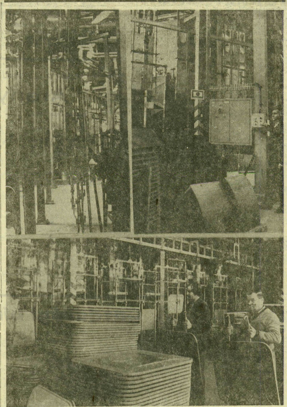
Gombnyomásra működő automata berendezés könnyíti a munkát az Ikarus szegedi gyárának festőüzemében. Két műszakban dolgoznak itt, naponta több ezer autóbuzs-alkatrész kerül a függő sín pályára. Zsírtalanító, alapozó, fényező és szárító egységeken át jutnak az elemek a szalag végére, ahol már csak csomagolásra, szállításra várnak.
