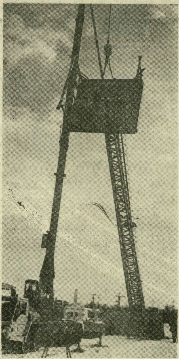
Somogyi Károlyné felvétele Világítótornyokat állítottak föl tegnap délelőtt a szegedi Városgazdálkodási Vállalat új forgalmi telepén. A három, egyenként harmincméteres torony tetején nagyfénerejű fényszórókat helyeznek majd el, amelyek az 5 hektáros munkahelyet kellőképpen megvilágítják.
