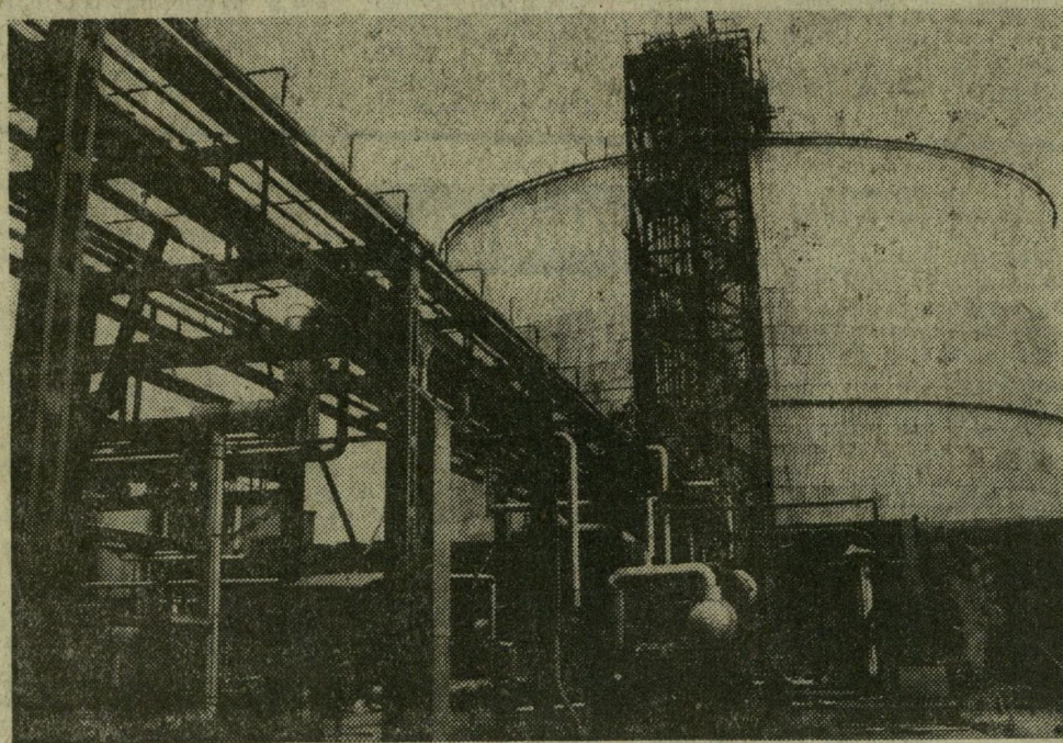
Elkészült az algyői olajmező leglátványosabb létesítménye, a 30 ezer köbméteres propán-bután tárolótartály. Ezekben a napokban már a próbaüzemelésre készítik elő, a benne levő levegő kiszorítása végett nitrogénnal öblítik át a szigetelt tartályt. A közeli napokban megérkeznek Budapestre a vezérlő programkártyák is, és sor kerülhet a komputer üzembe állítására. Felvételünk a hatalmas tartályról és kiszolgáló berendezéséről készült
