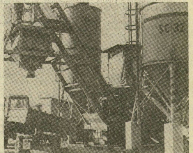
A betonkeverő a parkéni és temetői munkákhoz is szolgáltató építőanyagot
