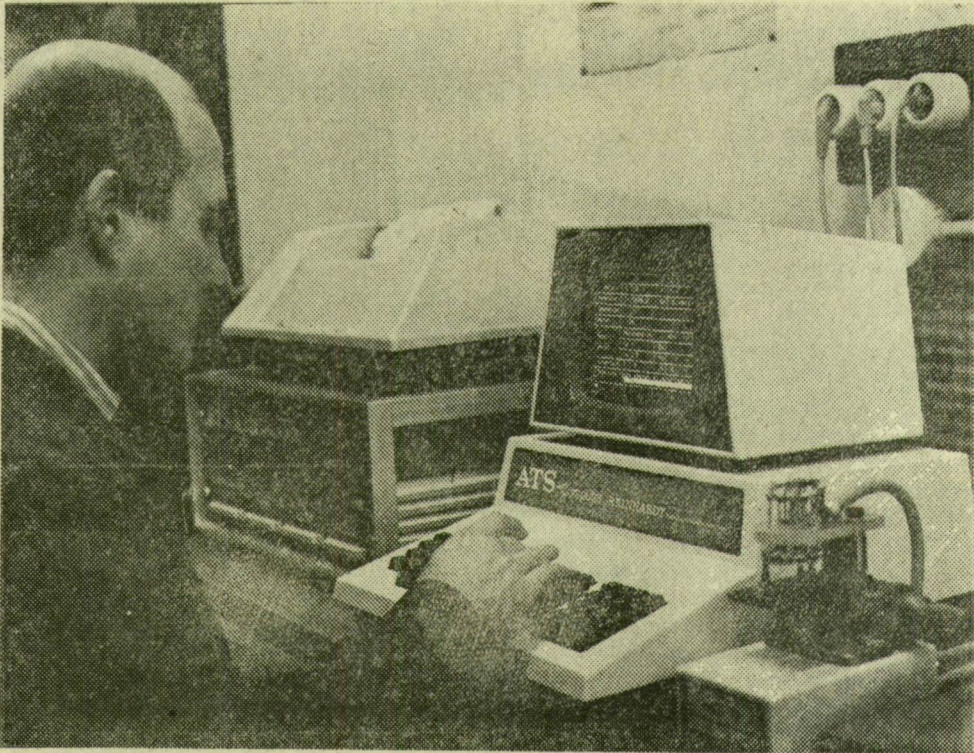
A REMIX Rádiótechnikai Vállalatnál több termék mellett úgynevezett szigetelő alapú vékony és vastag rétegáramköröket is gyártanak. Ezek rendkívül kicsik és alkalmazási területük sokrétű. A megrendelő kérésének megfelelően — egy-egy berendezéshez alakítva — készítik ezeket a speciális, miniatűr áramköröket, amelyek a távvezérlésben, az automatizálásban ma már nélkülözhetetlenek. A REMIX-nél tavaly nyolcvan-száz millió forint értékben készítették ilyen különleges mikroáramköröket. Képünkön: Krémer Péter nagy bonyolultságú hibrid áramkört ellen őriz.
