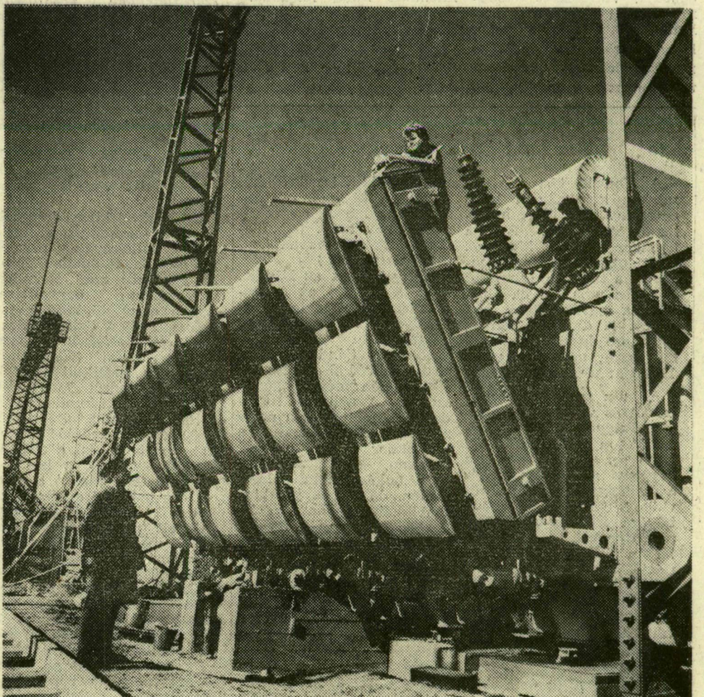
A Ganz-MÁVAG szerelői a transzformátorok beállításán dolgoznak
