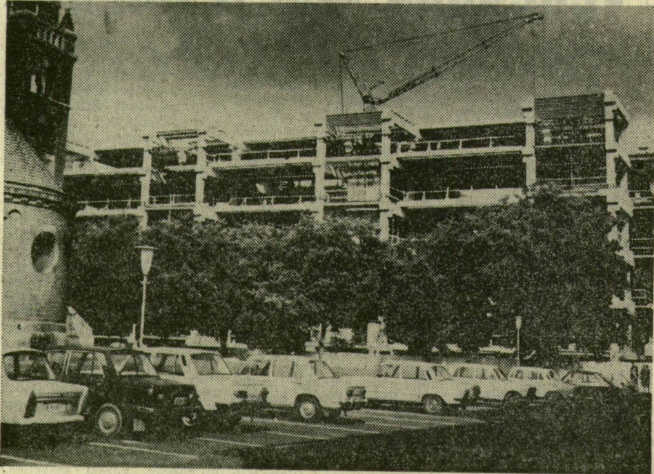
Teljes magasságában és végleges formájában mutatkozik már a Dóm téren épülő könyvtár. Az előre gyártott hatalmas vasbeton tartópillérek és földemelek összerakása hosszadalmas feladatot jelent, a DÉLÉP dolgozói ezekben a napokban is ezt a munkát végzik
