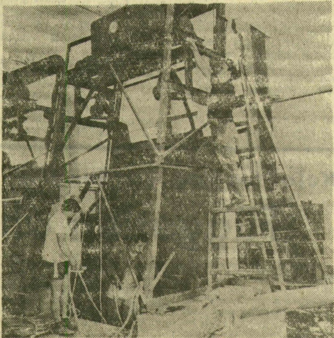
A megszürt szennyvízből a felfogott szerves törmelékelt a Geiger-rács segítségével távolítják el. Képünkön a kiemelőszerkezet szerelés közben.
