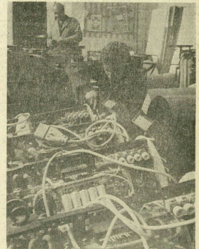
A VBKM Erősáramú Elektronikai Gyárának budafoki gyáregységében tirisztoros ivhegesztő berendezéseket készítenek. A szocialista piacon egyedülálló berendezéssel különleges minőségű követelményeknek is megfelelő varratot lehet készíteni, többek között ezért használják ezt a hegesztőgéptípust a Paksi Atomerőmű szerelési munkáinál is
