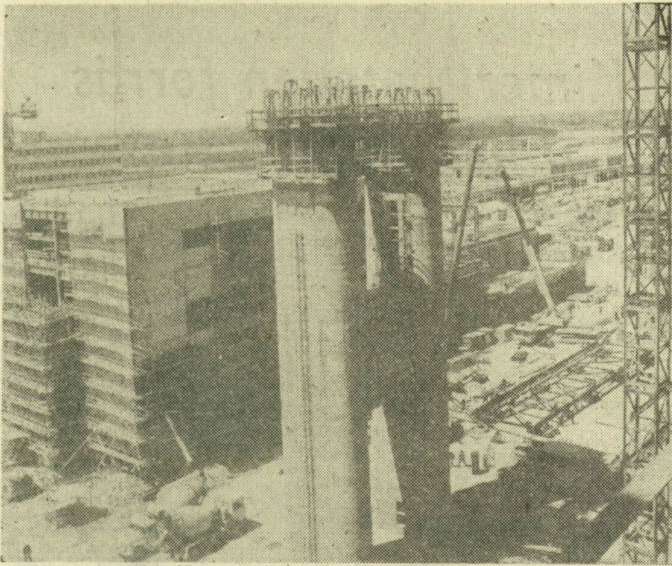
Az ítemtervnek megfelelően épül a Paksi Atomerőmű hatalmas és különleges kéménye
