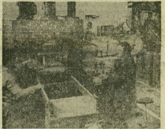
Roncsolásos próba a betonmintán
