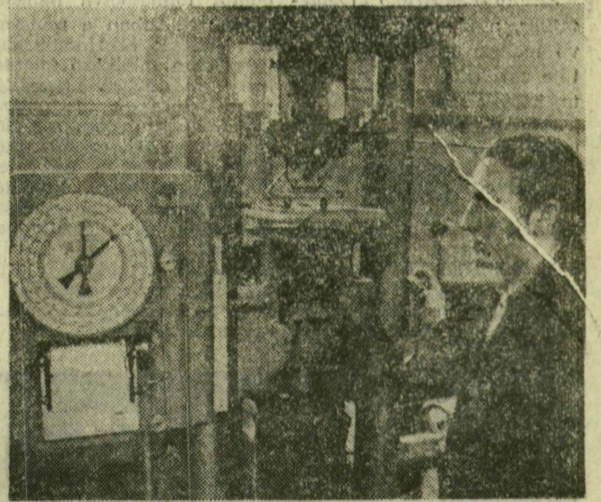
Műszer segítségével mérik a cserép hajlítószilárdságát
