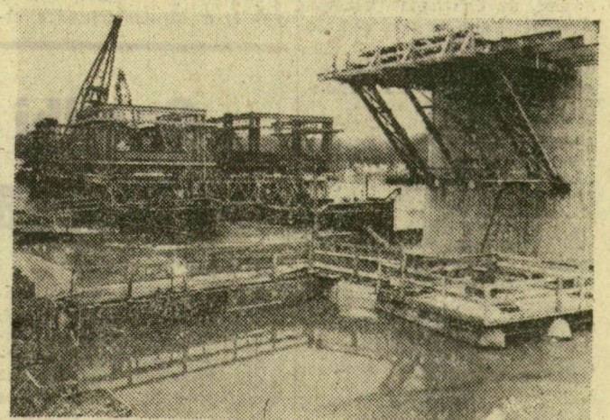
A Szentes felüli mederpillér mögött kataránra helyezve szerelték össze a szaluzókocsikat
