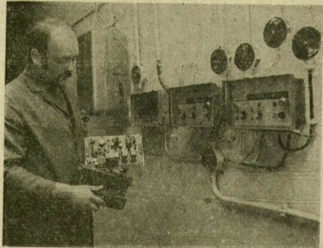
A Fővárosi Tűzfűtő Művek a fűtőenergia gazdaságosabb kihasználása érdekében a hőközpontokat fokozatosan felszereli fűtőszabályozókkal. E készülékek a külső hőmérséklet függvényében szabályozzák a lakásokba jutó fűtővíz hőfokát. Képfőképen: szerelik a fűtőszabályozó vezérlőegységét az egyik óbudai hőközpontban
