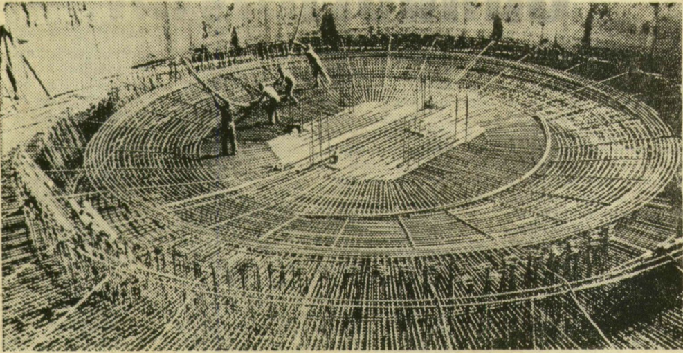
Készül a víztorony alapozásának beton vasszerkezete
