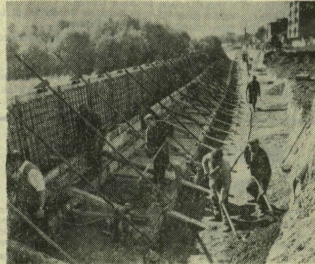
A mellvéd-falat betonozzák a Nacynilés Gáspár vezette szocialista brigád fagjai
