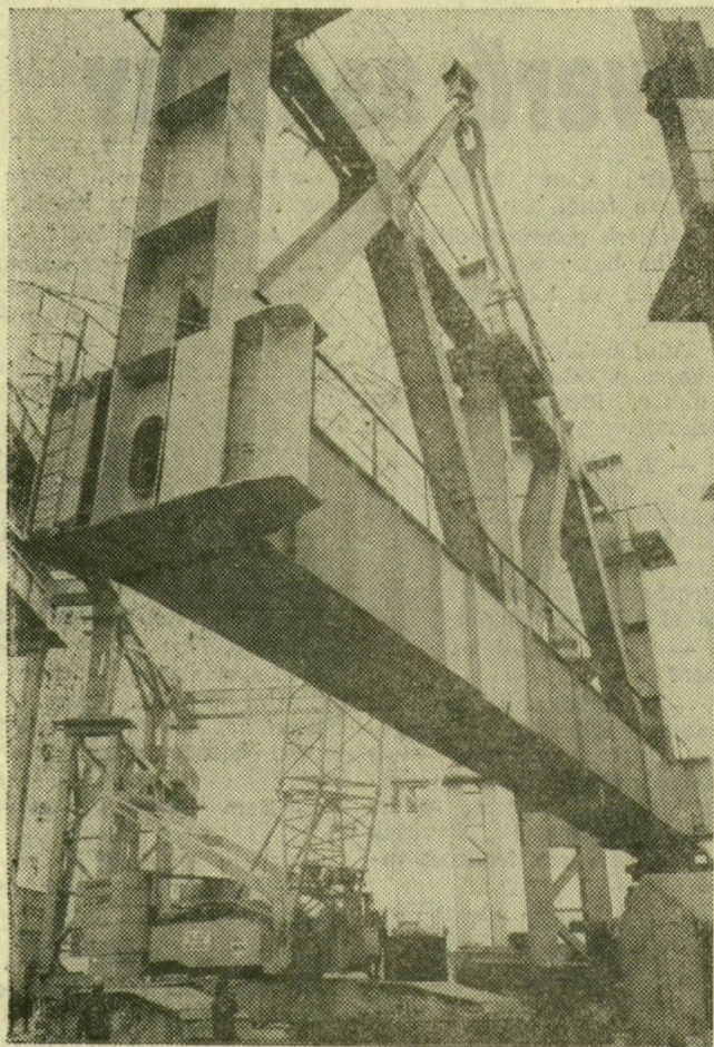
Dunaújvárosban, a Dunai Vasmű területén jó ütemben épül az új, konverteres acélmű, amely elkészülte után évente több mint egymillió tonna acélt fog előállítani. Most az építők a harminc méter magas oszlopok tetejére emelték a gyártócsarnok szízhétyven tonnás fő tartóelemét. A képen: Levegőben a súlyos teher. (MTI-fotó — KS)
