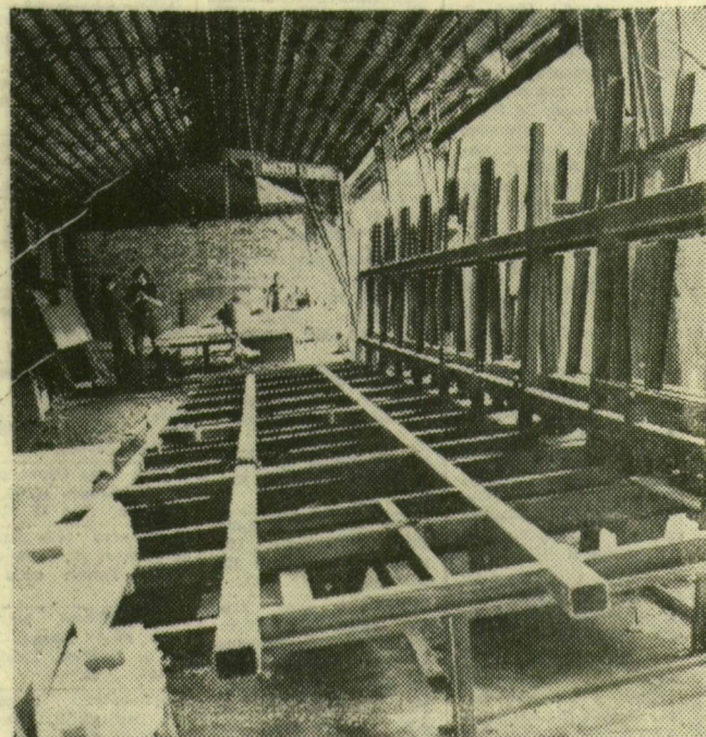
Néhány hónappal ezelőtti kép: ezekre a vashordákra kerülnek föl a 3 milliméteres krómácel lemezek
