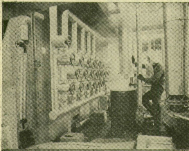
Leninvárosban üzembe helyezték a Tiszai Vegyi Kombinát hatodik termelőegységét, a polipropilengyárat, amely évente negyven ezer tonna polipropilén gyártására képes. A képen: mintavétel az oldószer-regenerálónál
