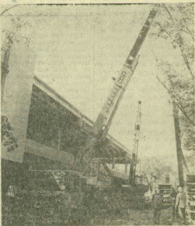
A homlokzati paneleket szerelik a Dugonics téren épülő Domus Áruházra a DÉLEP szakemberei. Japán gyártmányú, KATO autódaruval emelik helyére az öt, illetve hat tonna súlyú elemeket
