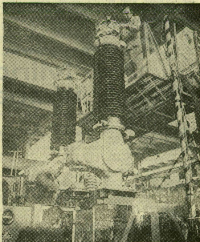
A Ganz Villamosági Művek óbudai gyárában nagyfeszültségű szakaszoló- és megszakító-berendezéseket gyártanak. A megszakítókat és a szakaszolókat elsősorban a hazai távvezeték- és erőműépítéseknek használják fel, de már szállították belőlük Peruba is. Képfőnök: A próbaterebben ellenőrzésre készülő elő a nagyfeszültségű megszakítókat
