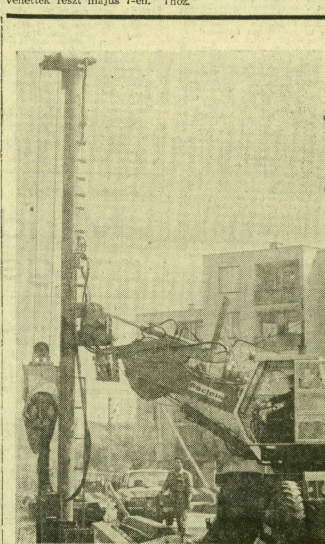
A Közmű- és Mélyépítő Vállalat új munkagépet állított üzembe. A cölöpverő és -kihúzó gép nem veri a cölöpöt a földbe, hanem valósággal „belerázza”. A vibrációs fej másodpercenként több ezres mozgását a cölöp átadja a homokszemcséknek és fellazítja a földet!
