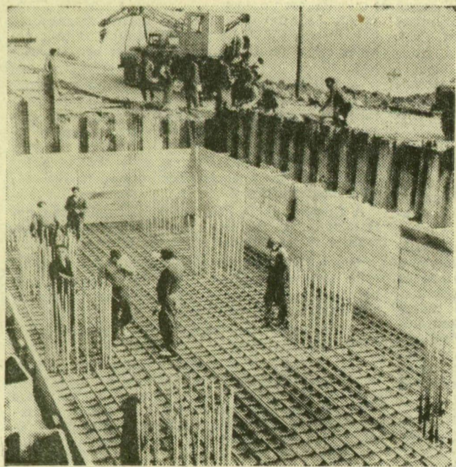
Szádfalak védelmében dolgoznak a betonacél-szerelők
