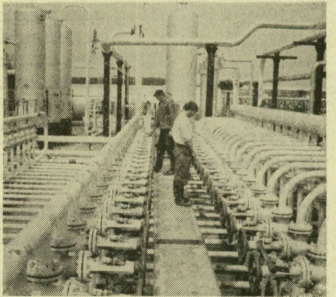
A zalai olajbányászat egyik legrégebbi lelőhelye a lovászi olajmező. A kimerülőben levő kutak „felélesztésére” új módszert honosítottak meg a Dél-dunántúli Köolaj- és Földgáztermelő Vállalat szakemberei: vizet és széndioxidgázt szajtolnak a kutakba. Az így keltett nyomás felszínre hozza az olajat. Az idén ezzel a módszerrel 9 ezer tonna olajat bányásznak. Képünkön: a fogadóállomás
