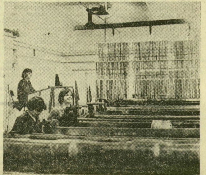
A galvanizálóüzemben gombnyomásra történik az anyagok mosatása, vegyi kezelése. Régebben kézzel, nehéz munkával végezték ezt a munkát
