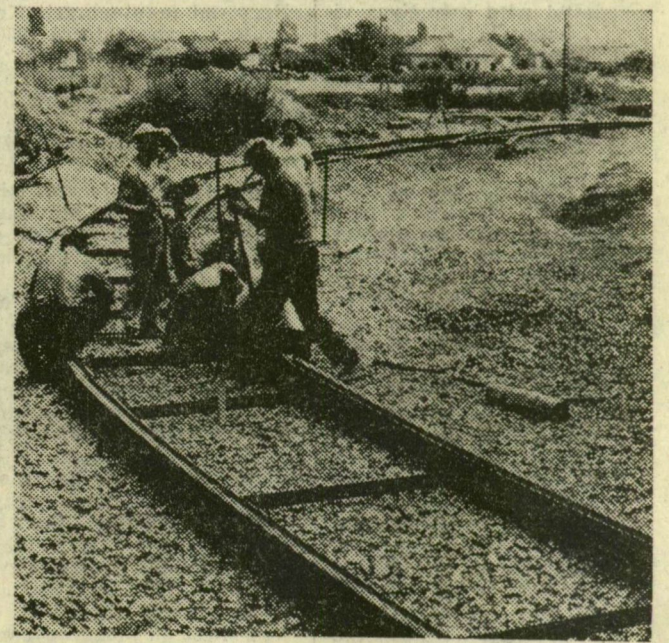
Somogyi Károlyné felvételei. Utasaikat letéve, itt, a feltöltött tavon fordulnak majd vissza a villamosok új pályájukra
