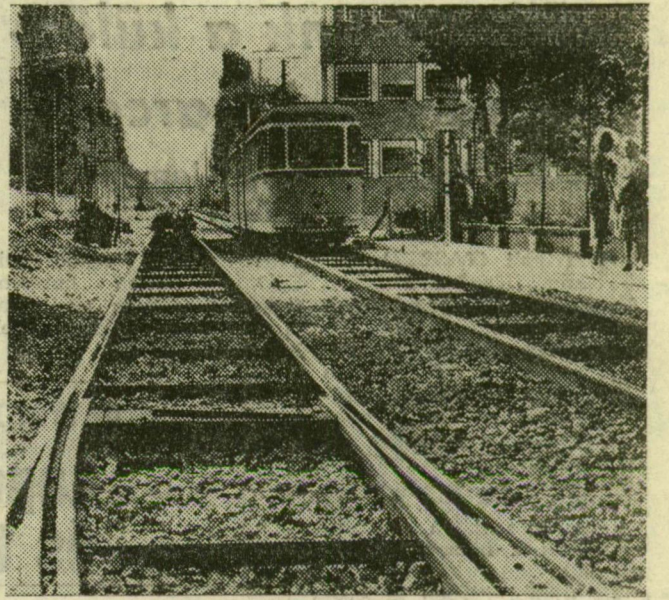
Az egyik sín kész a konzervgyár előtt, a másik már majdnem elkészült
