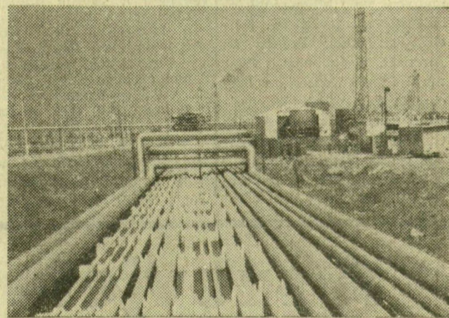
Leninvárosban hat és fél milliárd forintos beruházzal az év hárommillió tonna kőolaj feldolgozására alkalmas finomítót építenek. Jelenleg, a tartálypark kialakítása mellett, nagy ütemben halad a Szovjetunióból származó termelőberendezések szerelése, összeállítása és felállítása a helyszínen. Képünkön: az épülő üzem részlete
