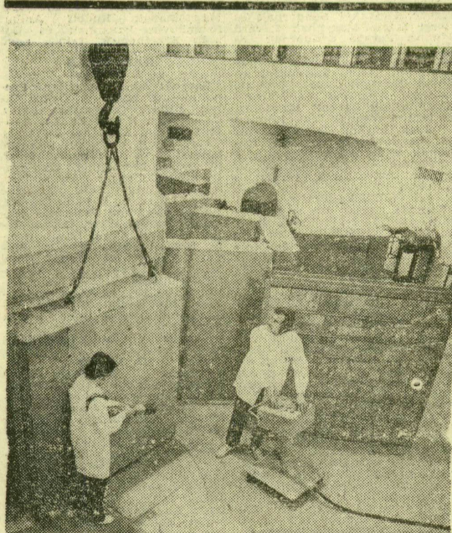
A Budapesti Műszaki Egyetem tanreaktorában különféle betonfajták sugárvédő tulajdonságait ellenőrzik, és kiválasztják a Paksi Atomerőmű reaktortömb építésére alkalmas típust. A tanreaktor munkatársai a nagy jelentőségű mérések alapján szakvéleményt adnak az atomerőmű tervezőinek.
