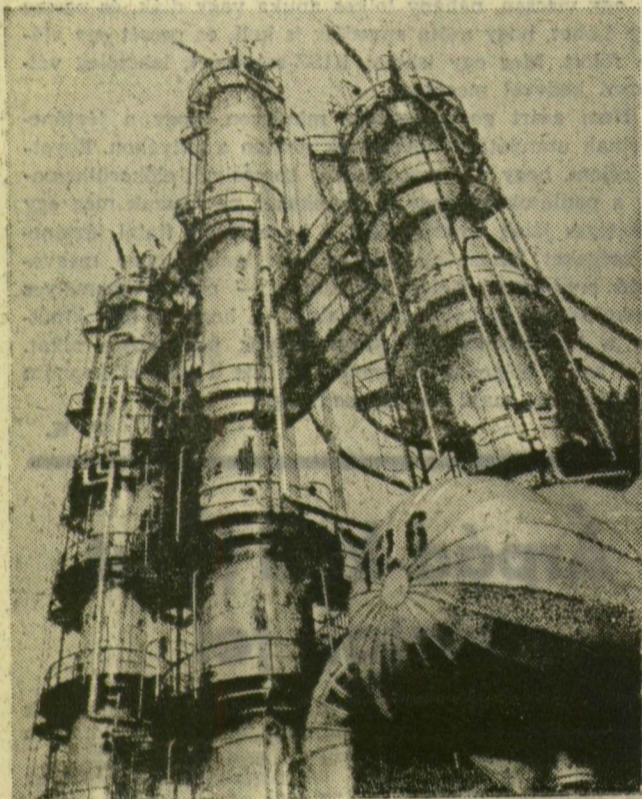
A Duna Kőolajipari Vállalat területén a tervezettnél korábban elkészült az új gázfrakcionáló üzem, amely évente 200 ezer tonna kőolajipari melléktermékből állít elő fűtőgázt, valamint cseppfolyós propán-pután gázt. Képünkön az üzem részlete.
