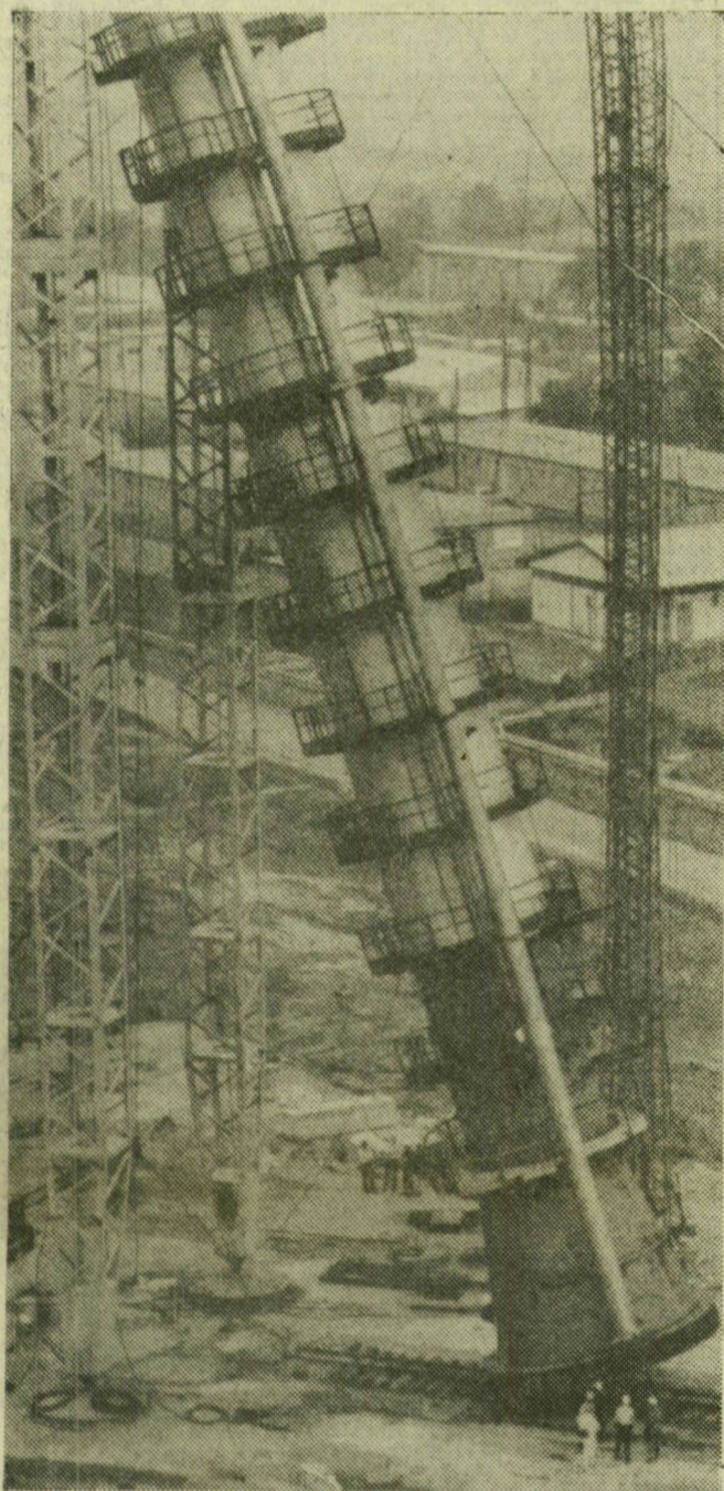
A Dunai Köolajipari Vállalat területén egy 400 tonnás, csaknem 80 méter magas desztilláló tornyot, több daru és csőrő segítségével állították a helyére. Képünkön: Az emelés
