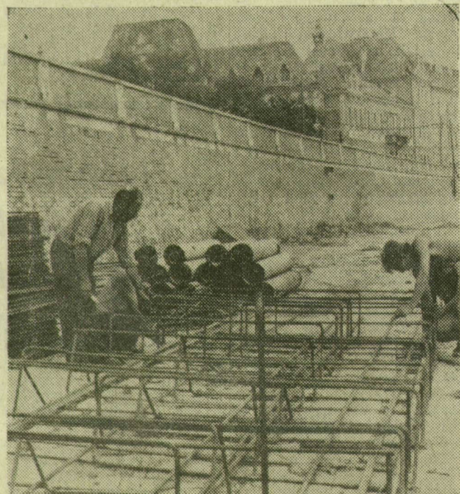
A VÍZÉP szakemberei készítik a pillérek acélszerkezetét
