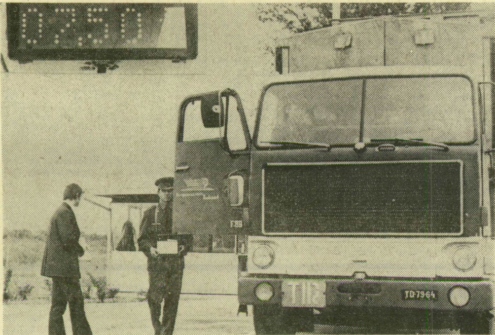
Mérik a Hungarokamion egyik kocsijának tengelysúlyát a rőszkei határállomáson. A Metripont által gyártott mérleg a pavilon falán levő kis táblán jelzi a súlyt
