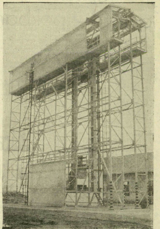
Pácsonyiban, a Szombathelyi MEZŐGÉP Tröszt 3. számú gyáregységében sorozatban gyártják már a hazai tervezésű, félautomatikus üzemi magasztárakat. A magasztárnak az az érdekessége, hogy az árut emeletesen tárolhatják, az anyagmozgatást pedig felvonóval oldották meg, látkép a magasztárról
