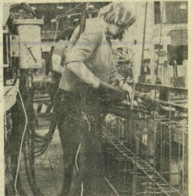
A panelek betonvasait ponthegező gépekkel állítják össze, s ezzel megadják a leendő szerkezet formáját is.
