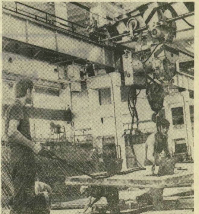
Acs S. Sándor felvétele! A gőzölőkamrában „érlelt” betonelemet daru segítségével szakítják ki a sablonból. Ezután már lehet szállítani az építkezéshez.
