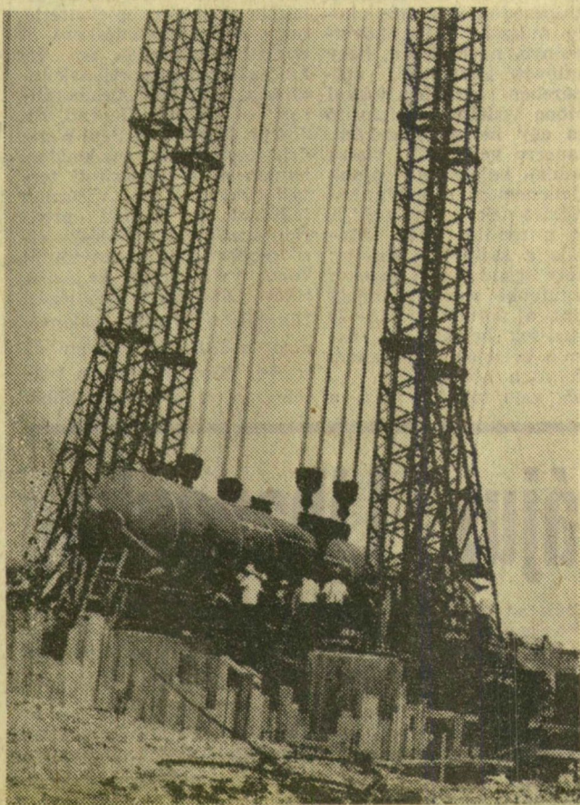
A gázüzem mellett újabb szovjet gyártmányú leparálótornyot helyeznek el az építők
