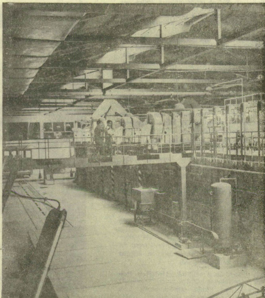
A SZENTESI TÉGLAGYÁR EGYIK GÉPSORA
