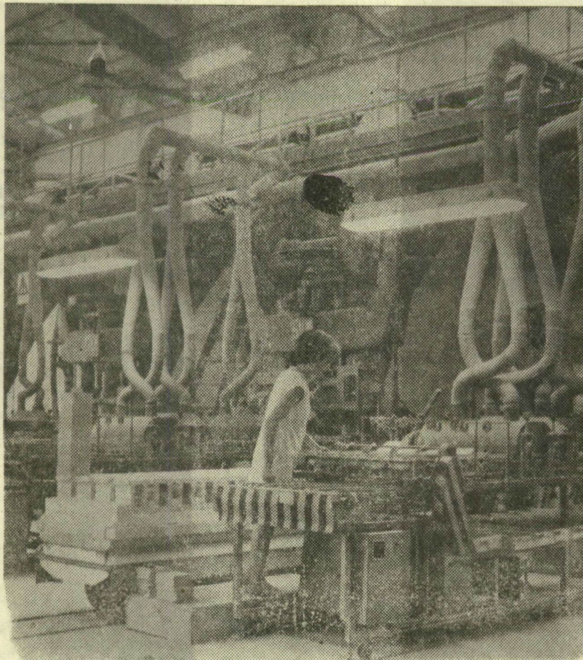
A FIM ALFÖLDI PORCELÁNGYÁRÁNAK CSEMPEGYÁRI PRÉSGÉPSORA
