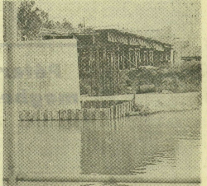
A Tisza jobb oldalán már elkezdték az úttest építéséhez szükséges kiegészítő acéltartók szerelését
