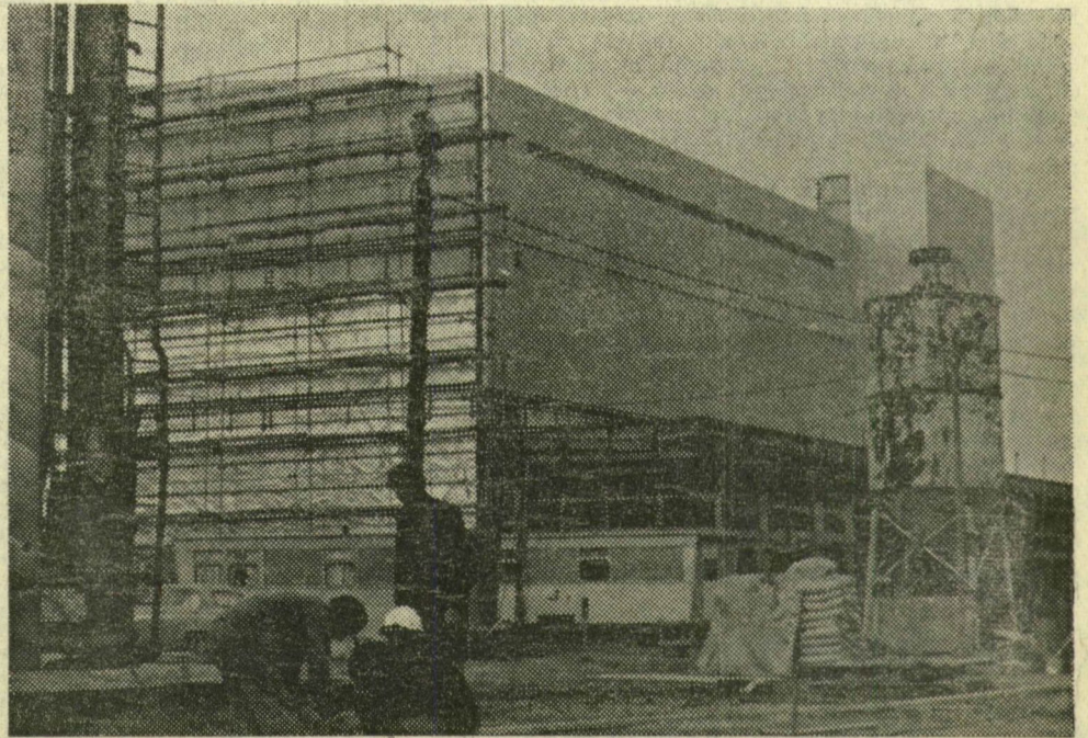
Az új hűtőház előtt — amelynek szigetelését és burkolását most végzik — elkészült az első mintacölöp. Képünk a DELEP cölöpverő berendezését mutatja munka közben
