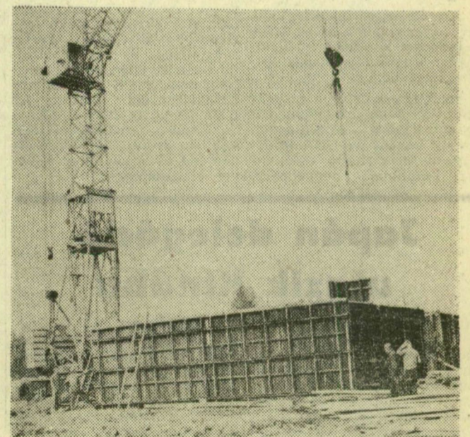
Acs S. Sándor felvételei. A résalapozás mellett, az 503-as épületet térszaluzással építik. Ennek a módszernek nagy előnye, hogy lényegesen meggyorsítja a munkát
