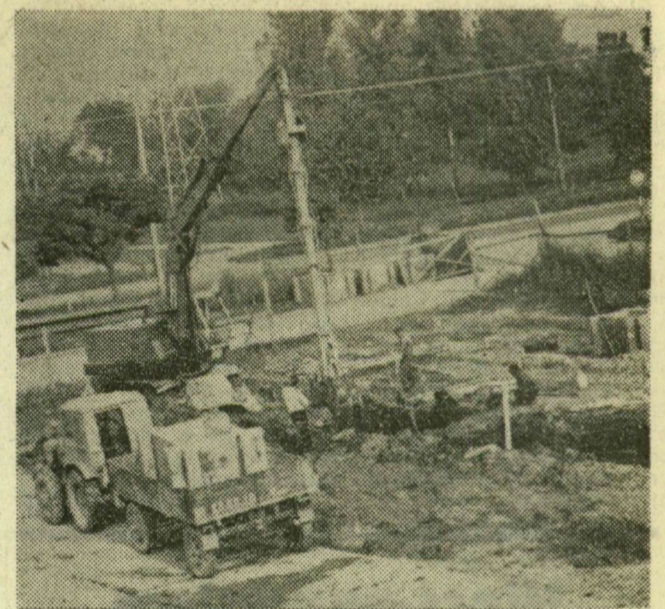
Közvetlenül a textiltechnikum mellett, 12 méter mély, ügynevezett résalapozással készül az 501 és 502-es jelű lakóház
