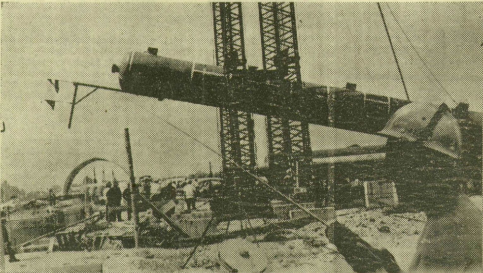
Az acéltornyó emelésének első pillanata. A százhusz tonna súly alatt megfeszülnek a drótkötelek
