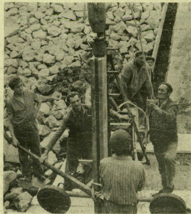
Cölöpverő dolgozik a mindszei szádfal építésénél
