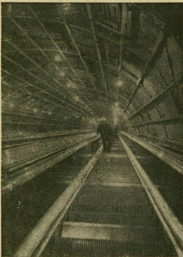
A metró második szakaszának Kossuth téri mélyalvó-másáról vezet a felszínre Budapest leghosszabb mozgólépcsője. A 70 méter hosszú szerkezet 34,80 méter mélyből szállítja majd a felszínre az utasokat. Az építők jól haladnak a munkálatokkal.
