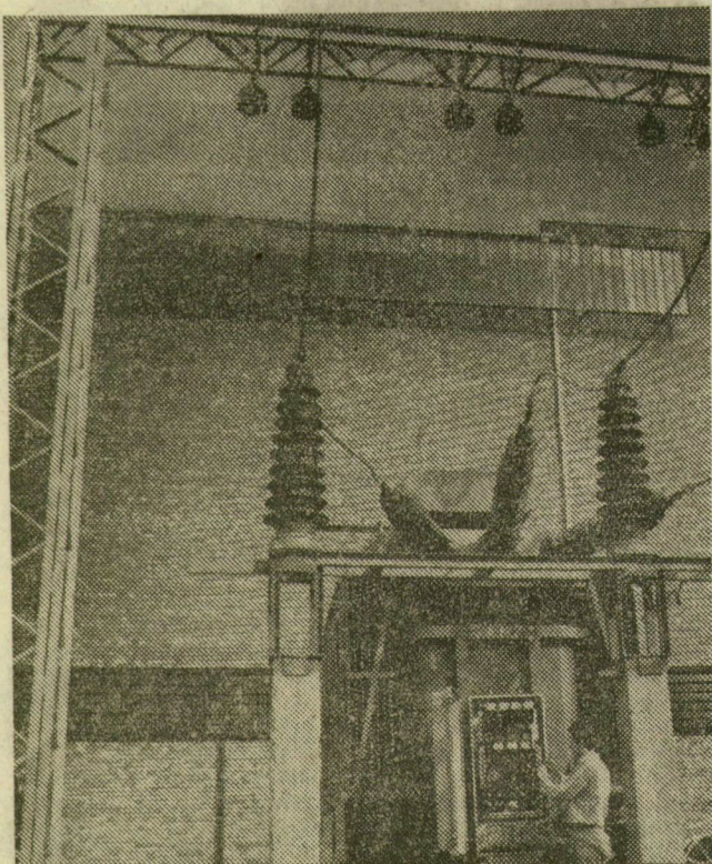
A trafóhoz itt csatlakozik a 100 kV-os nagyfeszültségű vezetékek
