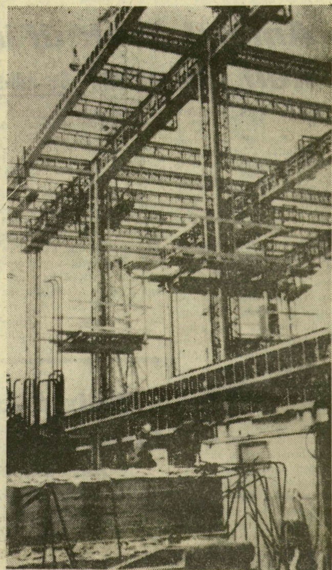
A már meglevő Dunai Hőerőmű szomszédságában az ediginél kétszer nagyobb teljesítményű erőművet építenek. A berendezések egy része csehszlovák, más része hazai gyárakban készül. Az erőmű 1976-ra épül fel. Generáltervezője az ERŐTERV, kivitelezője pedig a 22. számú és 26. számú Állami Építőipari Vállalat
