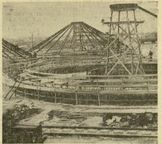
Somogyi Károlyné felvétele. A gyártócsarnok mögött épülnek a belonsílok. Az egyik silóépítmény szaluzását készítik
