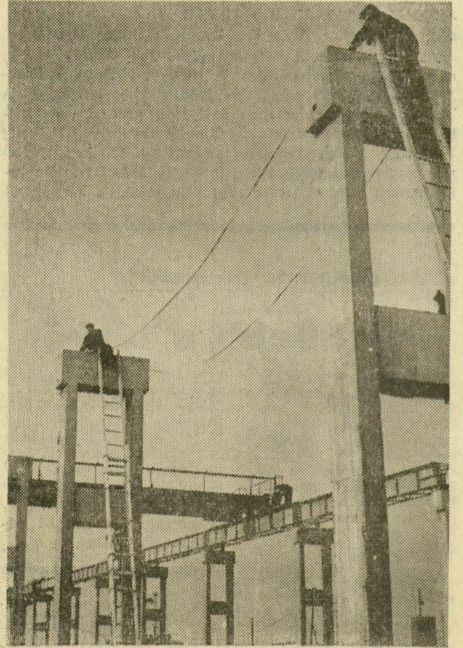
A csarnok főbejárata előtt, a vasbeton oszlopok tetején darupályákat képeznek ki
