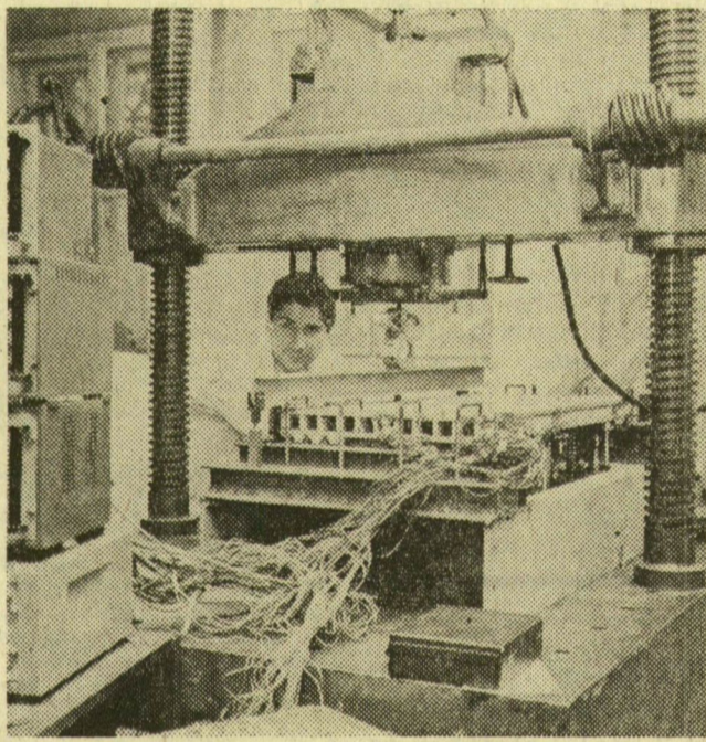
ERŐPRÓBA. A Budapesti Műszaki Egyetem acélszerkezeti tanszékén fontos kísérleteket folytatnak. Modelleken vizsgálják az egyes középületek, lakóházak, hidak szerkezeteinek terhelési viszonyait. A KPM megbízásából folytatott kísérletek célja az előregyártott közúti hidak leg-gazdaságosabb és erőjáték szempontjából kedvezőbb kiválasztása.
